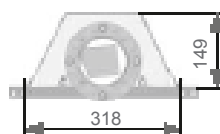
Doorsnede
